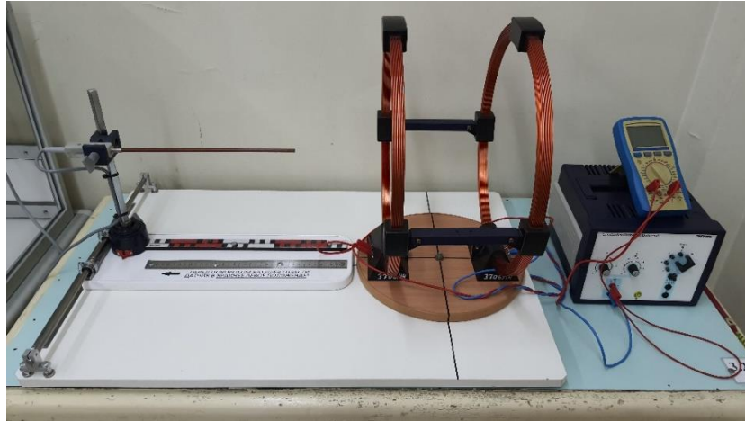
Рис. 2. Модернизированная установка для изучения свойств магнитного поля
