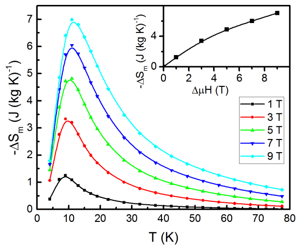
Рис. 2 Магнитокалорический эффект NdRh_2 для разных изменений поля \Delta\mu_0 H = 1, 3, 5, 7 и 9 Т. На вставке рисунка – зависимость максимума эффекта от поля.
