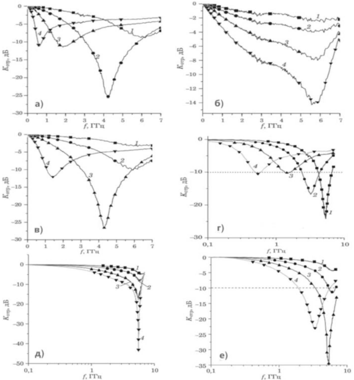
Рисунок 1. Частотные спектры коэффициента отражения K_{\text{отр}} композитов Ф2М/Mn-Zn (а), Ф2М/Ni-Zn (б), Ф42/2000HM (в), Ф42/2000HN (г) (концентрация — 20 (1), 40 (2), 60 (3), 80% (4)), ПС525/Mn-Zn (д), Ф2М/ LiMnZn (е), (концентрация 9 (1), 21 (2), 37 (3), 61% (4))
