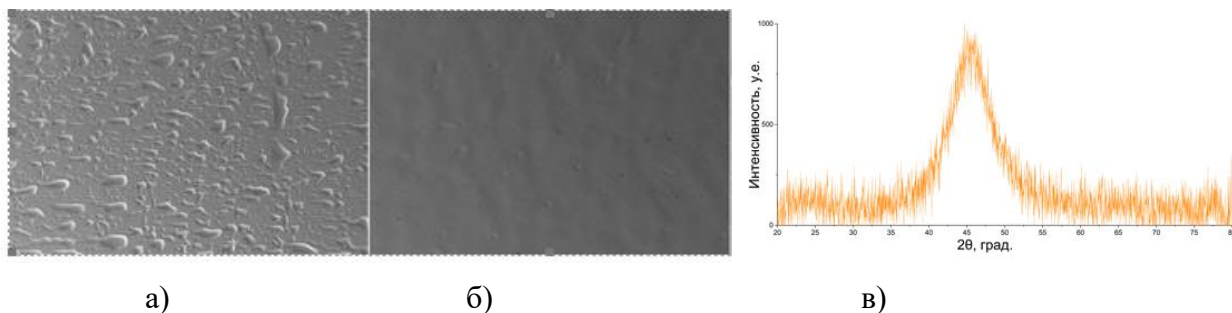
Рис. 2. Электронно – микроскопические изображения (а) контактной поверхности; (б) свободной поверхности; (в) профиль рентгенограммы быстрозакаленного сплава Fe-Co-Ni-Si-B
