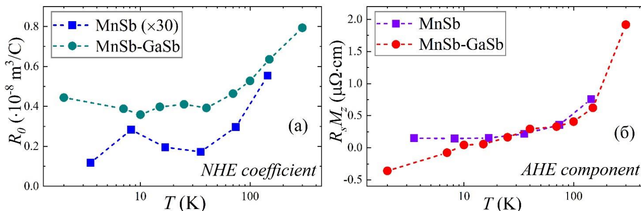
Рис. 2. Температурная зависимость (а) коэффициента нормального эффекта Холла R_0 и (б) амплитуды аномального эффекта Холла для исследуемых образцов. Значения R_0 для кристалла MnSb были умножены на 30 для большей иллюстративности.
