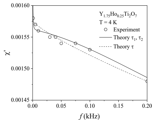
Рис. 2. Результаты аппроксимации частотной зависимости динамической АС восприимчивости для допированного титаната гольмия Y_{1.75}Ho_{0.25}Ti_2O_7 для температуры 4 К
