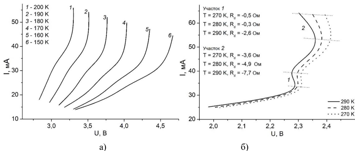
Рис. 2. Вольт-амперные характеристики образцов манганитов: La_{0.7}Sr_{0.3}Mn_{0.9}Fe_{0.05}Sc_{0.05}O_{3+\gamma} , отожженного при P_{O_2} = 10^5 Па (а); La_{0.7}Sr_{0.3}Mn_{0.9}Fe_{0.05}Co_{0.05}O_{3+\gamma} , отожженного при P_{O_2} = 10^{-1} Па, в магнитном поле (б)
