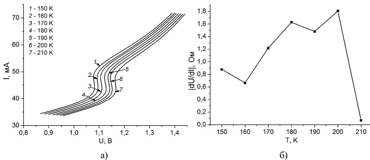
Рис. 2. Вольт-амперные характеристики при различных температурах (а) и температурная зависимость максимального модуля отрицательного дифференциального сопротивления (б) образца манганита, отожженного при P_{O_2} = 10^5 Па
