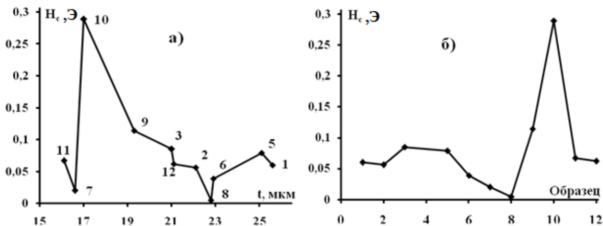
Рис. 5. Изменение коэрцитивной силы: а) в зависимости от толщины образцов (цифры – номера образцов); б) в зависимости от режима получения
