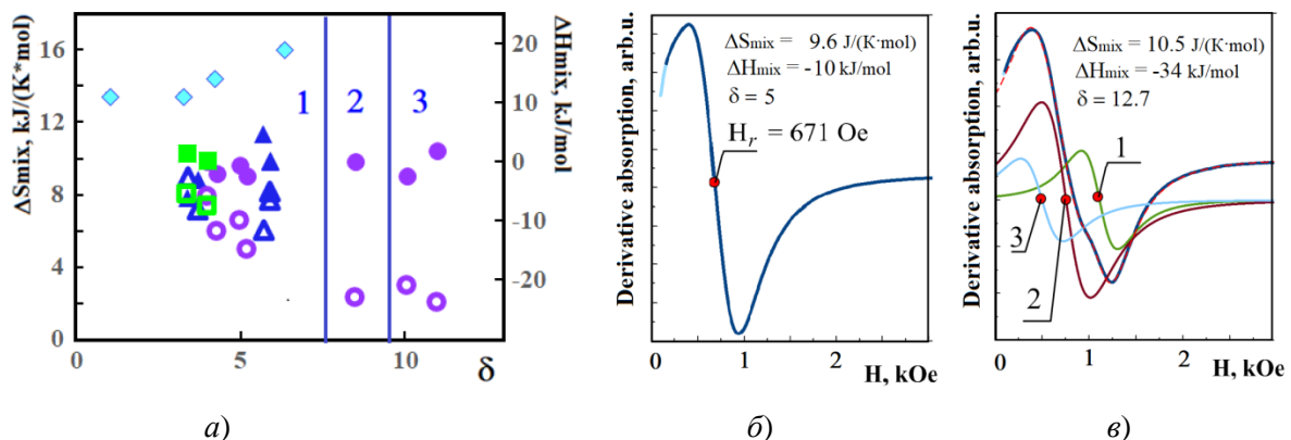
Рис. 1. Влияние основных факторов \Delta S_{\text{mix}} (заполненные символы), \Delta H_{\text{mix}} (незаполненные символы), на фазовый состав покрытий из ВЭС (а). Треугольники - серия А, кружки - серия В, квадраты - серия С, ромбы данные работы [2]. Спектры ФМР в параллельной геометрии эксперимента для пленок \text{FeCoNiP-Zr} с различным содержанием Zr: (б)-2% Zr - однофазная пленка, (в)-20% Zr- многофазный сплав (приведен результат разложения спектра ФМР на парциальные лоренцианы)
