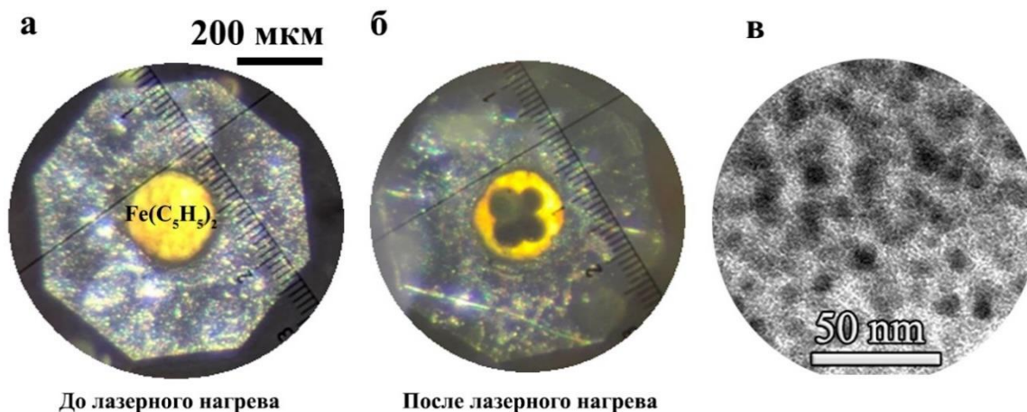
Рис. 1. Оптические фотографии калетты алмазной наковальни и ферроцена Fe(C_5H_5)_2 до (а) и после (б) лазерного нагрева. (в) ПЭМ изображение наночастиц, полученных в процессе превращений ферроцена при ВДВТ.
