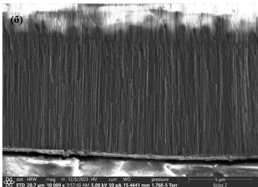
Рис. 1. Изображение растровой электронной микроскопии Co нанопроволок на сколе оксидной матрицы
