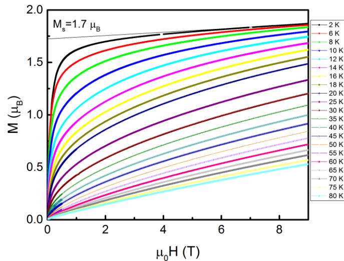
Рис. 1 Полевые зависимости намагниченности M(\mu_0 H) NdRh_2 для ряда температур в диапазоне 2 \leq T \leq 80 К.
