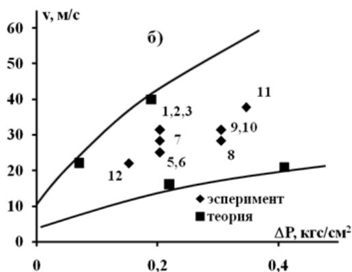
Рис. 1. Область значений линейной скорости закалочного диска и избыточного давления, обеспечивающих получение аморфных лент в исходном состоянии (цифрами обозначены номера плавок при различных значениях v и \Delta P )
