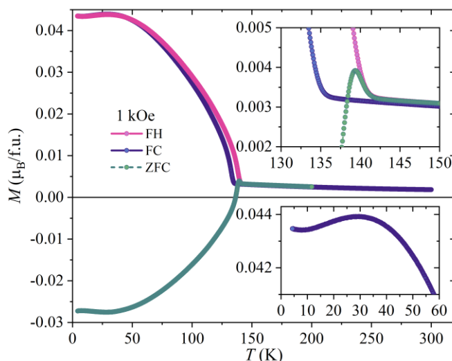
Рис.2 - Температурные зависимости намагниченности \text{Ni}_2\text{CrVO}_5 , измеренные в режимах с нулевым охлаждением (ZFC), полевом охлаждением (FC) и полевом нагревом (FH), H = 1 \text{ кЭ} . Верхняя вставка: увеличенный масштаб кривых M(T) вблизи магнитного перехода T_N . Нижняя вставка: куполообразная аномалия намагниченности (FC).
