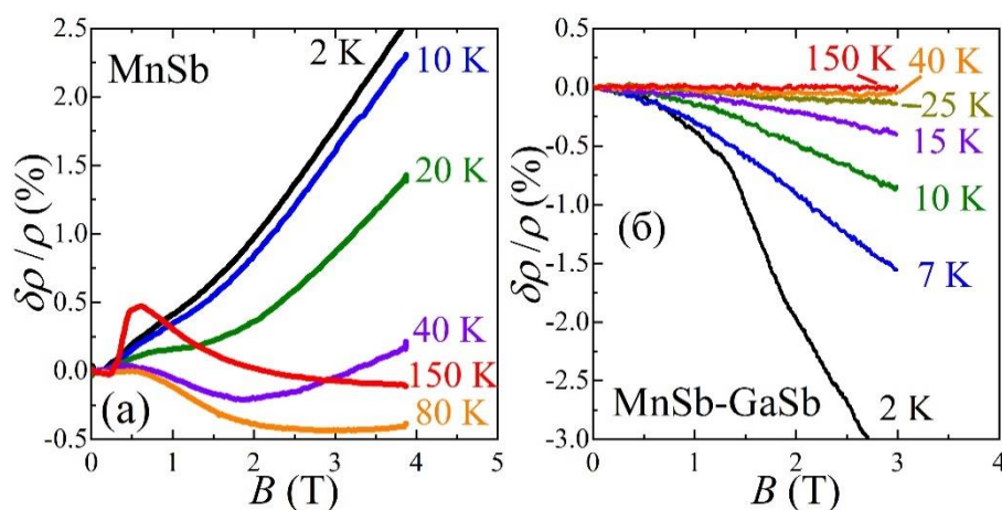
Рис. 1. Кривые магнетосопротивления при различных температурах для (а) кристалла MnSb и (б) композита MnSb-GaSb.
