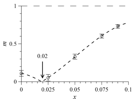
Рис. 3. Концентрационные зависимости параметра ангармонизма m в мультиферроиках \text{Bi}_{1-x}\text{Nd}_x\text{FeO}_3 при 295 К.
