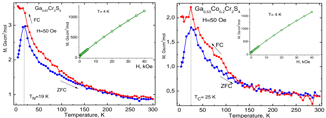
Рис. 2. Температурные зависимости намагниченности Ga_{2/3(1-x)}Co_xCr_2S_4 . На вставке: Полевые зависимости намагниченности.
