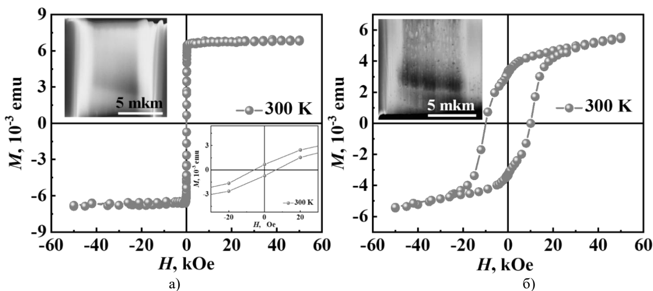
Рис. 1. Гистерезис намагничивания микропровода 1 до отжига (а) и микропровода 2 после вакуумного отжига (б). На вставках (а) и (б) показаны изображения ламелей микропроводов 1 и 2 соответственно, полученные в сканирующем электронном микроскопе
