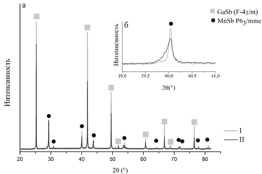
Рис. 1 (а) Рентгенограмма образца состава 59 мол% GaSb – 41 мол% MnSb: (I) v_{(охл)} = 0.1 о/с, (II) v_{(охл)} = 60 °/с.; (б) увеличенный фрагмент в области 40 град. 2\theta
