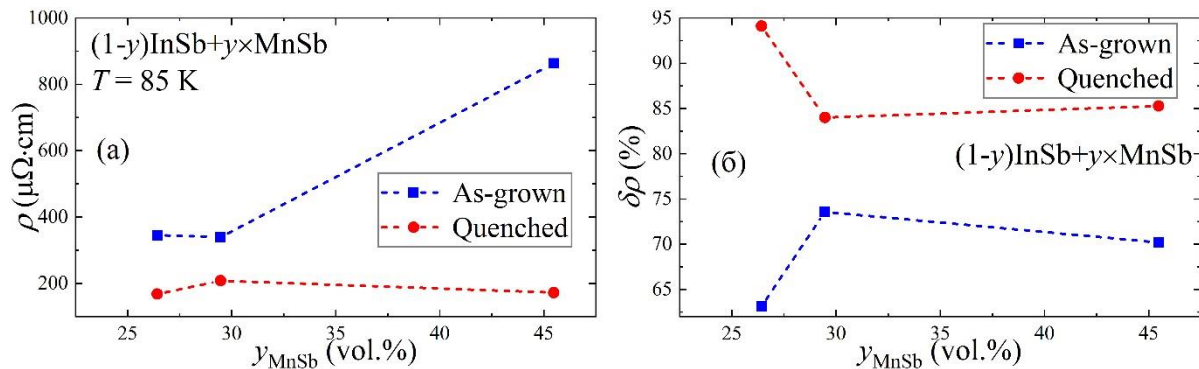
Рис. 2. (а) Композиционная зависимость удельного сопротивления закалённых и равновесных кристаллов InSb-MnSb при температуре 85 К; (б) композиционная зависимость относительной амплитуды изменения сопротивления \delta\rho с температурой для исследуемых образцов.
