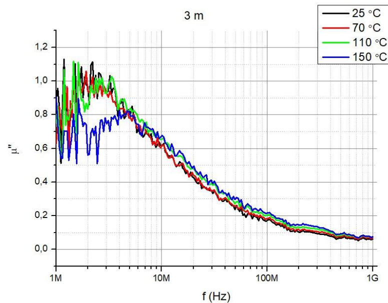
Рисунок 1 – График зависимости мнимой части магнитной проницаемости микропровода от частоты до отжига
