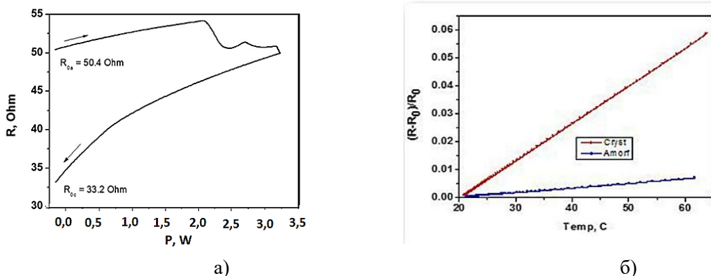
Рис. 1. Зависимость сопротивления от мощности R(P) (а); зависимость относительного изменения сопротивления микропровода от температуры в аморфном (синяя ветвь) и в кристаллизованном состоянии (красная ветвь) (б)
