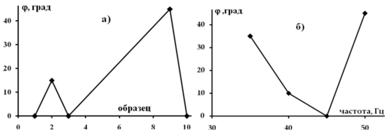
Рис. 4. Изменение угла анизотропии: а) в зависимости от номера плавки, для частоты 50 Гц ( v = 31,4 м/с) и б) в зависимости от частоты, для фиксированного давления в камере
