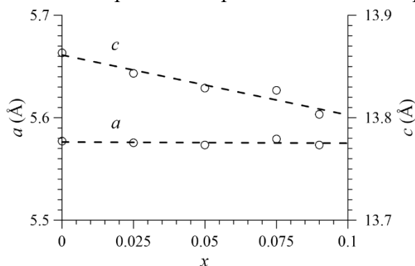
Рис. 1. Концентрационные зависимости параметров решетки исследуемых ферритов.
