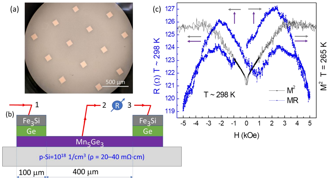
Рис. 1. Оптическое (а) и схематическое (б) изображение структур Fe_3Si/Ge/Mn_5Ge_3 . (с) Полевые зависимости электросопротивления R (левая панель) и квадрата намагниченности M^2 (правая панель) при температуре ниже T_C для Mn_5Ge_3 . Стрелками схематично показаны преимущественные ориентации вектора намагниченности ферромагнитных слоев структуры.
