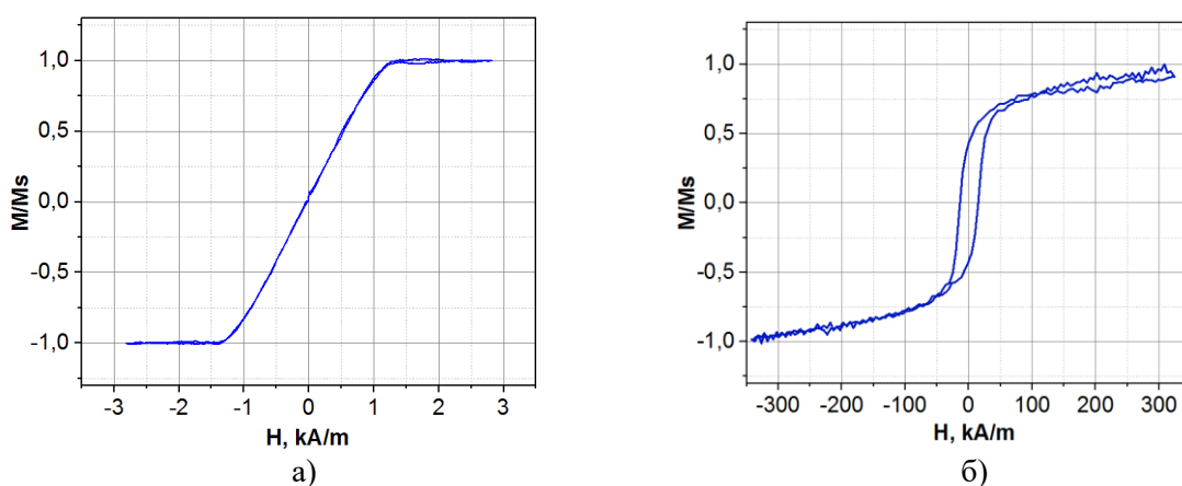
Рис. 2. Петля гистерезиса микропровода в исходном аморфном состоянии (а); петля гистерезиса микропровода в кристаллизованном состоянии после термообработки постоянным током (б)
