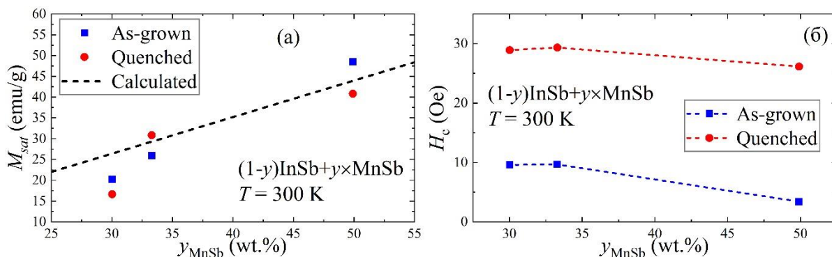
Рис. 1. (а) Композиционная зависимость намагниченности насыщения закалённых ( quenched ) и равновесных ( as-grown ) кристаллов InSb-MnSb при комнатной температуре; пунктирной линией показана расчётная зависимость отклика на основе литературных данных [1]; (б) композиционная зависимость коэрцитивной силы исследуемых образцов.
