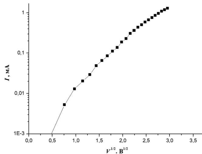
Рис. 2 Зависимость силы тока I от V^{1/2} при толщине DLC(Fe) 50 нм и концентрации Fe 20 ат.%.
