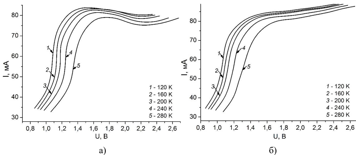
Рис. 1. Вольт-амперные характеристики исходного образца манганита при различных температурах: а – в отсутствие магнитного поля; б – в магнитном поле 0,92 Тл
