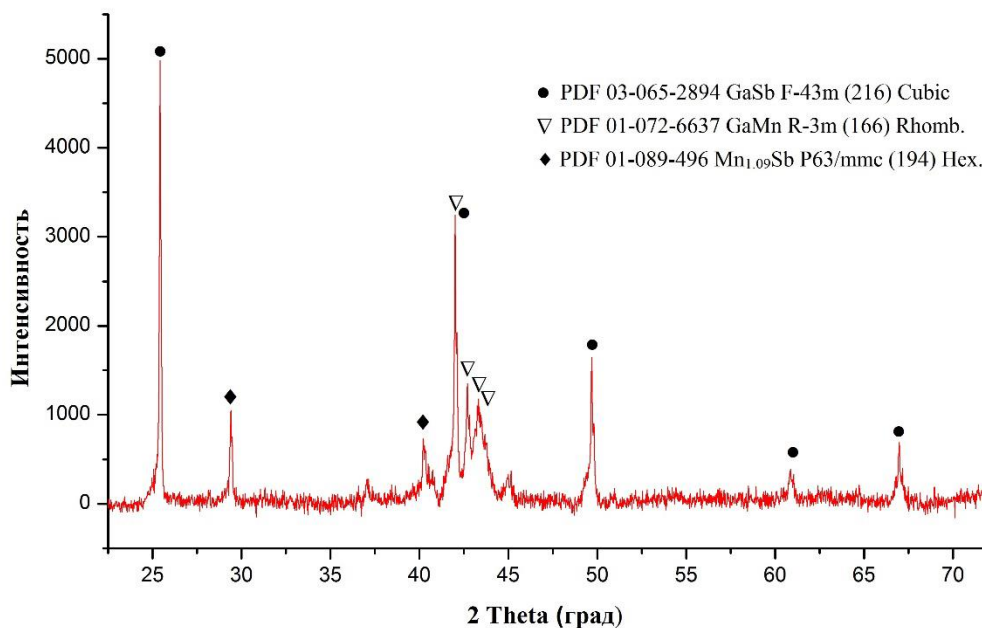
Рис.3 Дифракционная картина полученного композита GaSb-MnSb-GaMn
