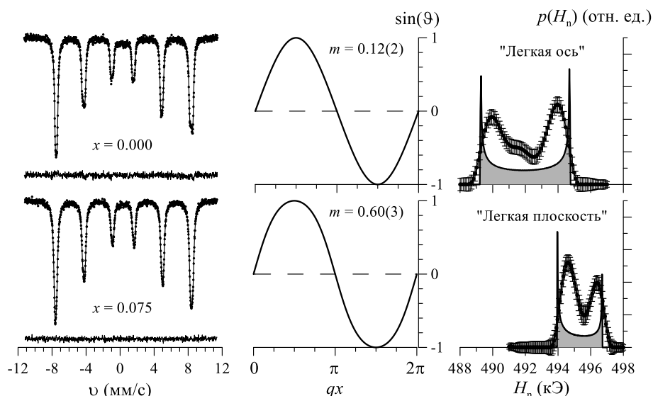
Рис. 2. Мессбауэровские спектры ядер ^{57}\text{Fe} в мультиферроиках \text{BiFeO}_3 и \text{Bi}_{0.0925}\text{Nd}_{0.075}\text{FeO}_3 и результаты их обработки в рамках модели АСМ циклоидального типа.
