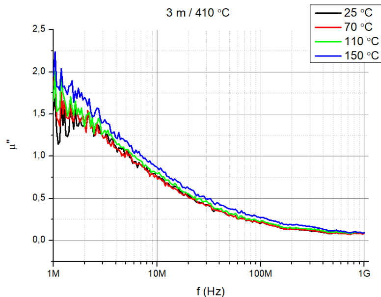
Рисунок 2 – График зависимости мнимой части магнитной проницаемости от частоты микропровода после отжига при 410 °C
