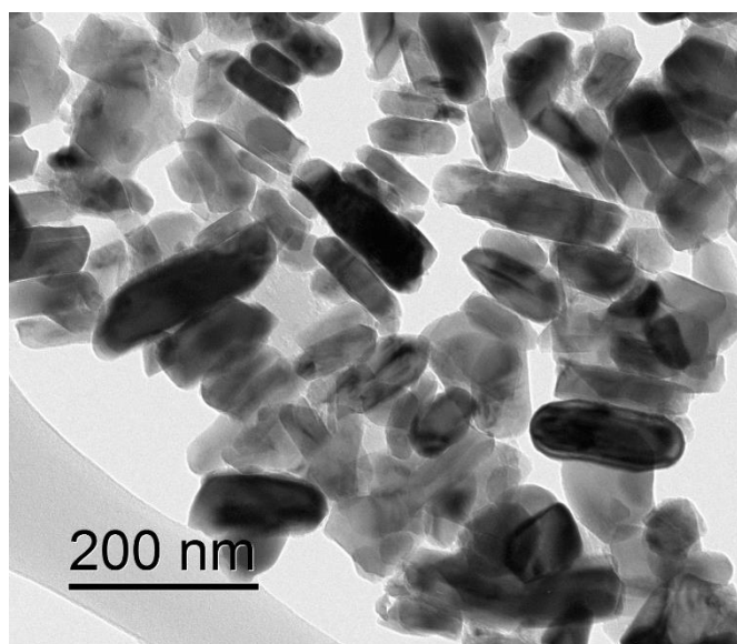
Рис. 2. Электронная микрофотография частиц \text{BaFe}_{12}\text{O}_{19}
