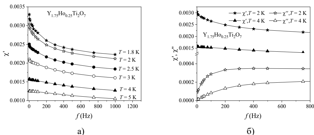
Рис. 1. \chi'_{\text{AC}}(f) , измеренная при температурах от 1.8 до 5 К (а); \chi'_{\text{AC}}(f) и \chi''_{\text{AC}}(f) , измеренные при температурах 2 и 4 К (б)
