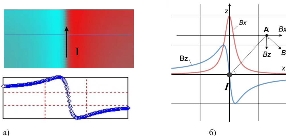
Рис. 2. Магнитное изображение вертикальной компоненты магнитного поля и поперечный скан, полученные с помощью сканирующего ГМИ-магнитометра (а); расчетные графики компонент вектора индукции магнитного поля над бесконечно длинным проводника с током (б)
