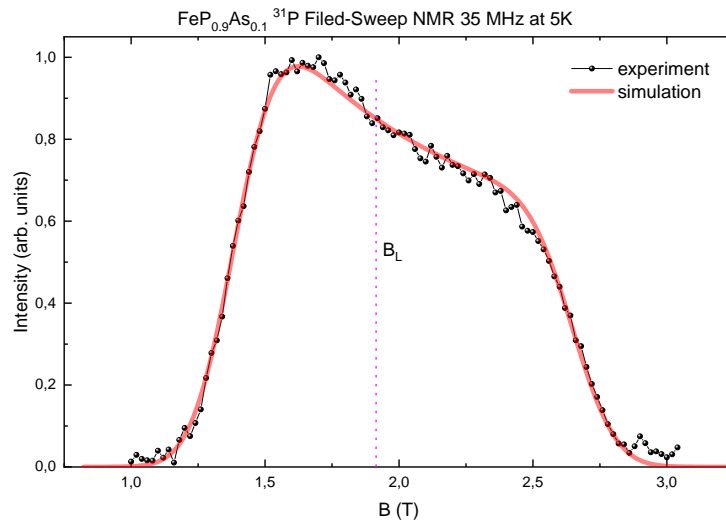
Рис. 1. ЯМР спектр FeP_{0.9}As_{0.1} на ядрах ^{31}P , снятый на фиксированной частоте 35 МГц. Черные точки – экспериментальные данные, красная кривая – симуляция, фиолетовая пунктирная прямая – Ларморовское поле ^{31}P на данной частоте.
