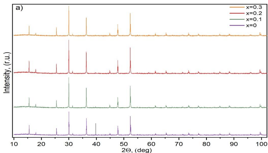
Рис. 1. Дифрактограммы твердого раствора \text{Ga}_{2/3(1-x)}\text{Co}_x\text{Cr}_2\text{S}_4
