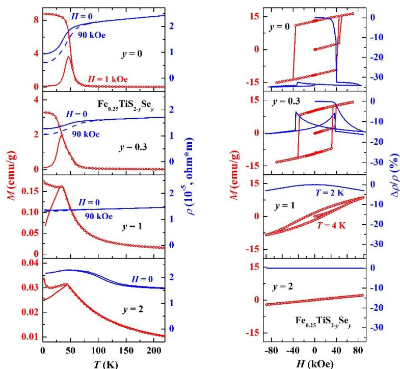
Рис. 1. Температурные зависимости намагниченности и электросопротивления (слева) и полевые зависимости намагниченности и магнитосопротивления (справа) для соединений \text{Fe}_{0.25}\text{TiS}_{2-y}\text{Se}_y с разным содержанием селена.
