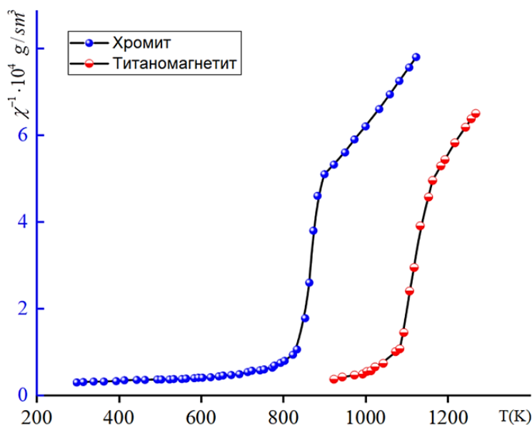
Рис. 1. Зависимости изученных образцов хромита – \text{FeCr}_2\text{O}_4 и титаномагнетита – \text{TiFe}_2\text{O}_4 .
