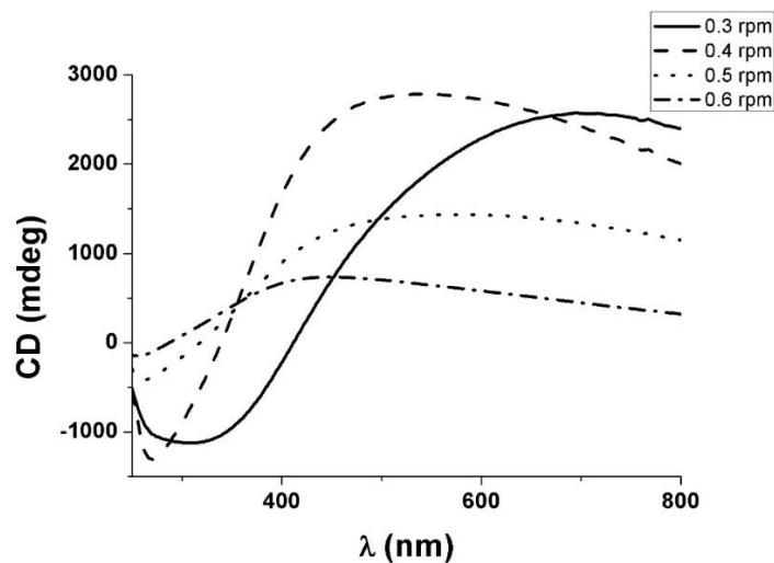
Рис. 2. Спектры циркулярного дихроизма (CD) для образцов, полученных при разных скоростях вращения подложки (0.3-0.6 об/мин).
