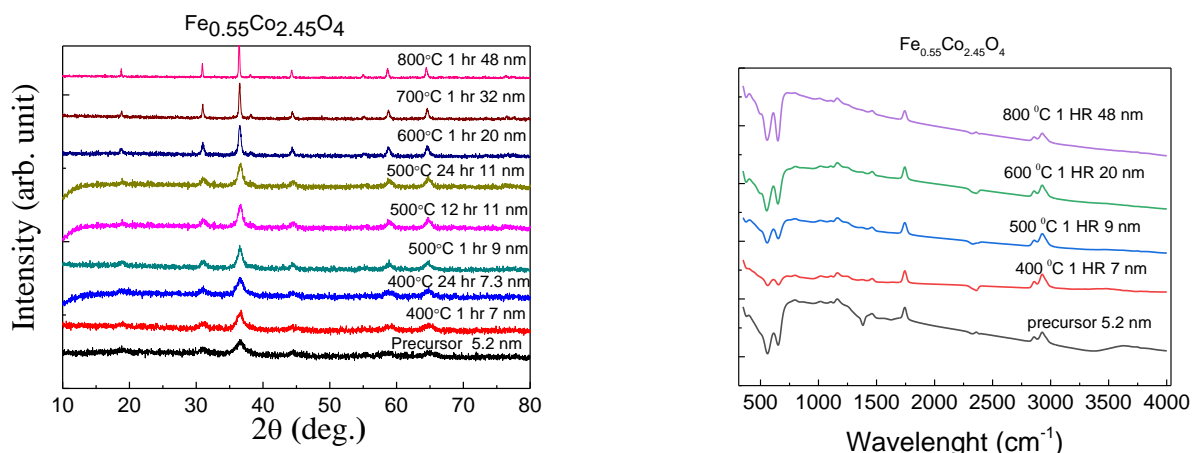
Рис. 1. Рентгеновские дифрактограммы (слева) и Фурье трансформанты ИК спектров (справа) исходного порошка НЧ (precursor) и после термообработки в различных режимах.
