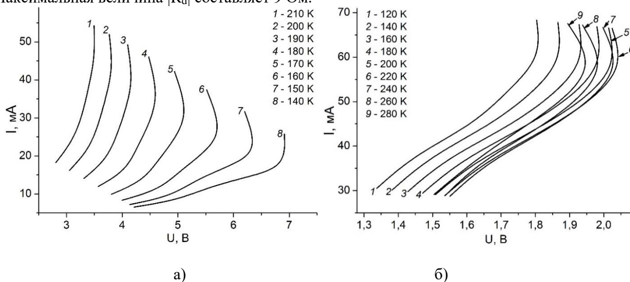
Рис. 1. Вольт-амперные характеристики манганитов La_{0.7}Sr_{0.3}Mn_{0.9}Fe_{0.05}Sc_{0.05}O_{3+\gamma} (а) и La_{0.7}Sr_{0.3}Mn_{0.9}Fe_{0.05}Co_{0.05}O_{3+\gamma} (б), отожженных при P_{O_2} = 10^{-8} Па
