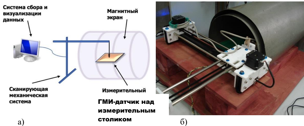
Рис. 1. Функциональная схема ГМИ-магнитометра (а); фотография лабораторного макета сканирующего ГМИ-магнитометра (б)
