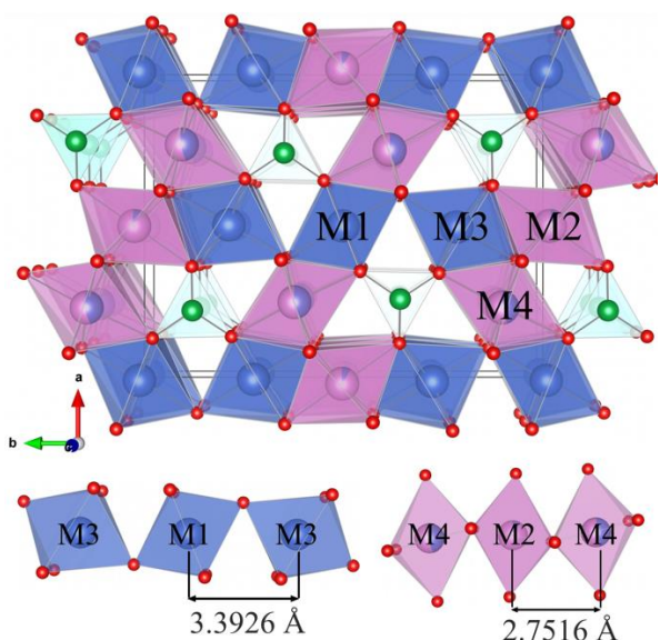
Рис.1 - Кристаллическая структура \text{Ni}_2\text{CrVO}_5 ( ab -плоскость) - два типа триад выделены синим и розовым цветом. Бор-кислородные треугольники показаны зеленым цветом. Внизу показаны самые длинные и самые короткие межионные расстояния в триадах M3-M1-M3 и M4-M2-M4, соответственно
