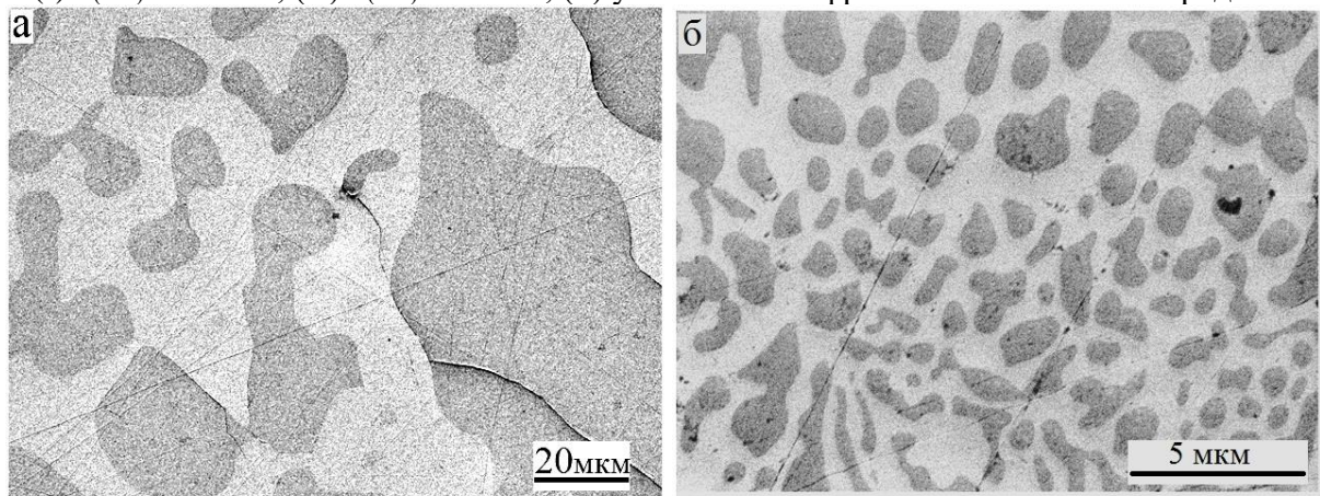
Рис. 2 (а, б) Микроструктуры образцов состава 59 мол% GaSb – 41 мол% MnSb: а) при v_{(охл)} = 0.1 °/с б) при v_{(охл)} = 60 °/с
