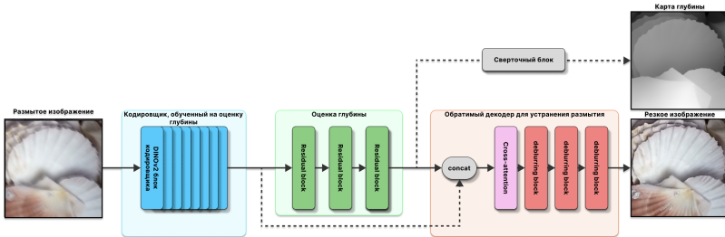
Рис 1. Общая схема предлагаемого метода RADBlur.
