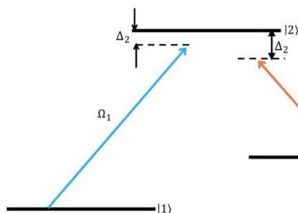
Рис. 1.1 Трехуровневая система активации лазерных импульсов
